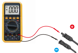
Figura 3.22 Medición del multímetro
