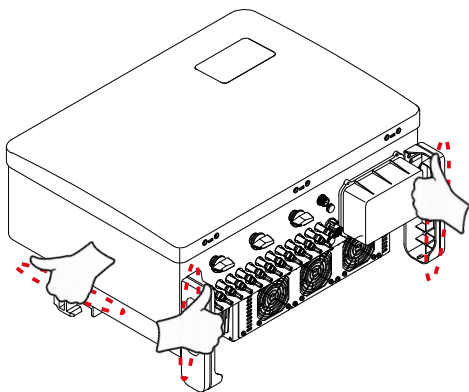
Figura 3.4 Manijas del inversor
